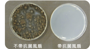
黑麴黴 NBRC 105649
